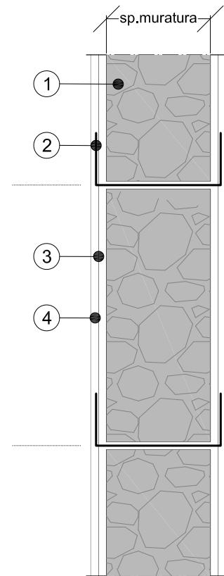
SEZ. B-B'
