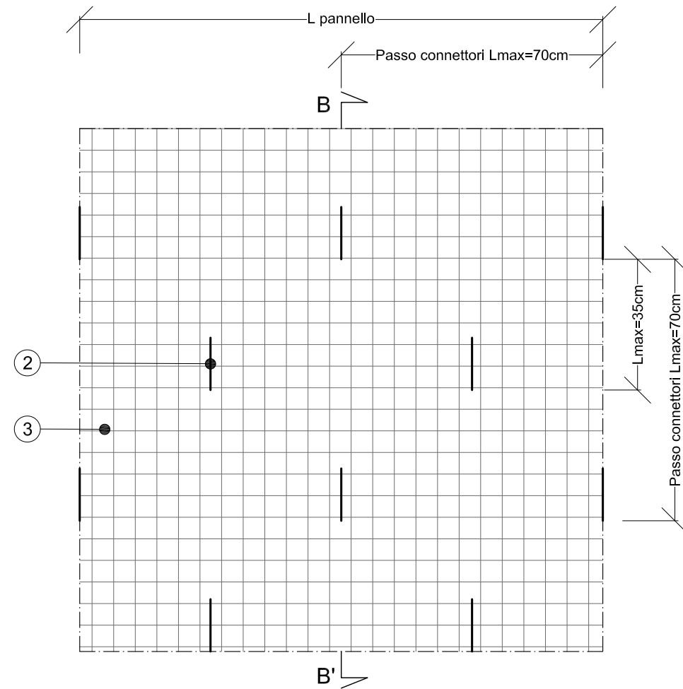
Prospecto della muratura rinforzata
