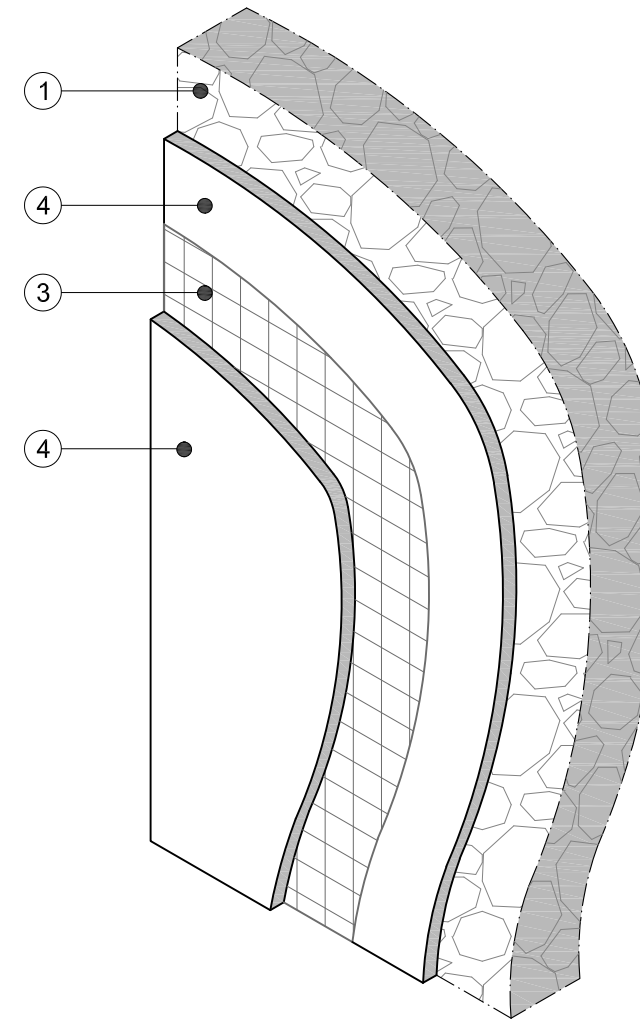
Assonometria
