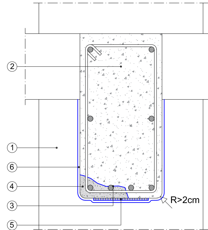
SEZIONE A-A'
