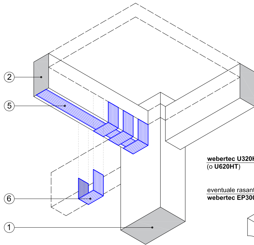
VISTA ASSONOMETRICA
