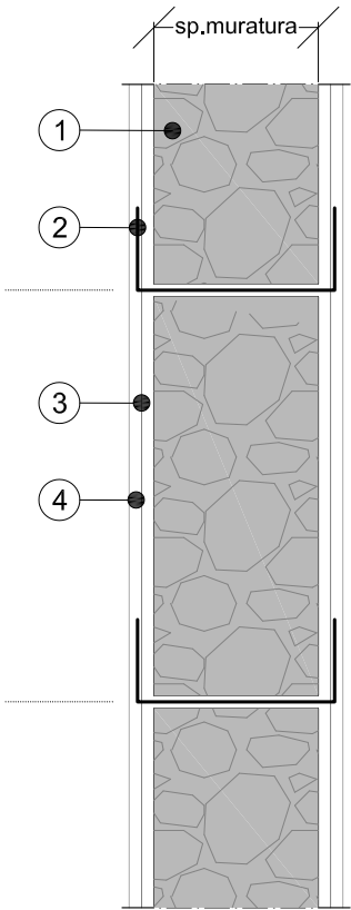
SEZ. B-B'
