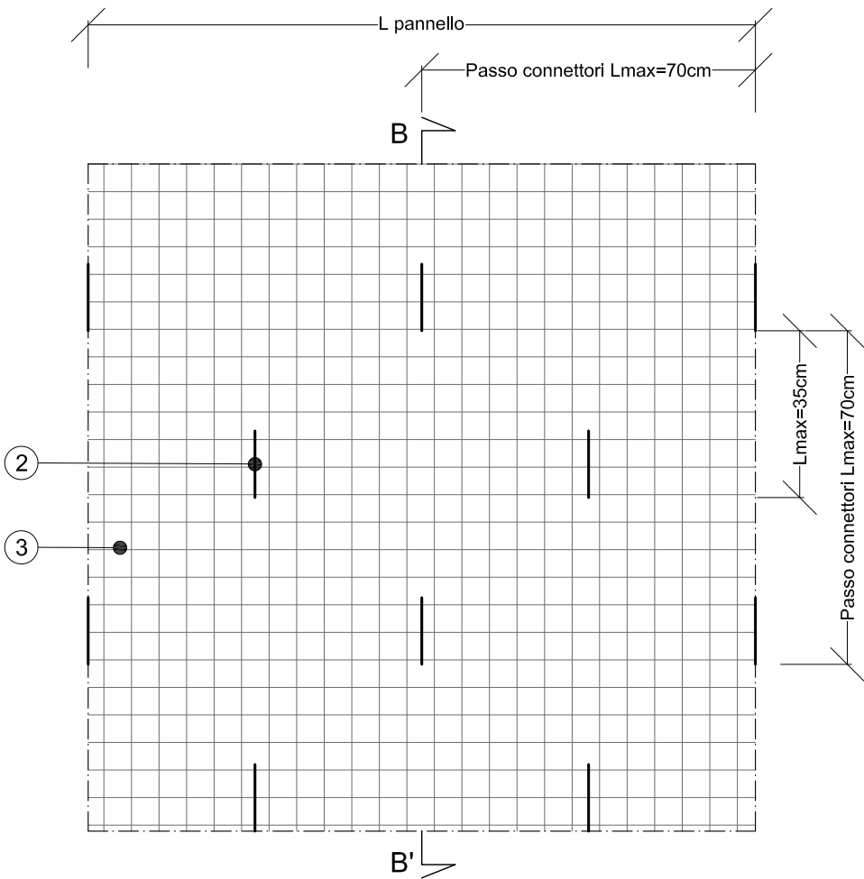
Prospetto della muratura rinforzata
