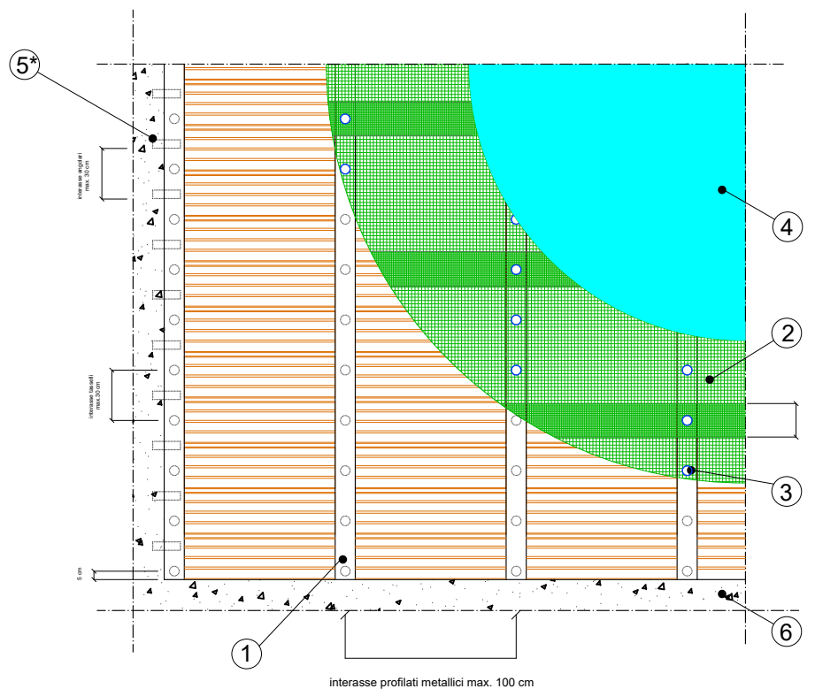
Pianta intradosso solaio
