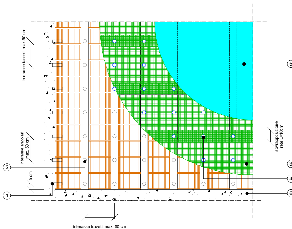
Pianta intradosso solaio
